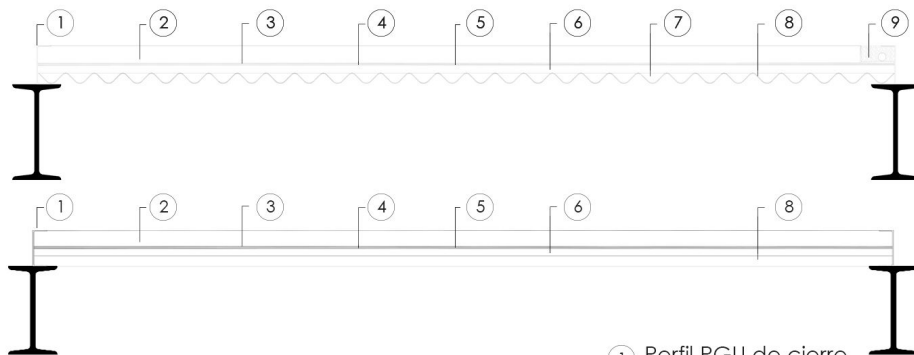
MÓDULO 4,5x4,5M: TECHO DE CHAPA
