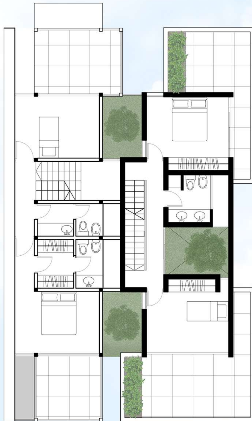
SEGUNDO PISO
