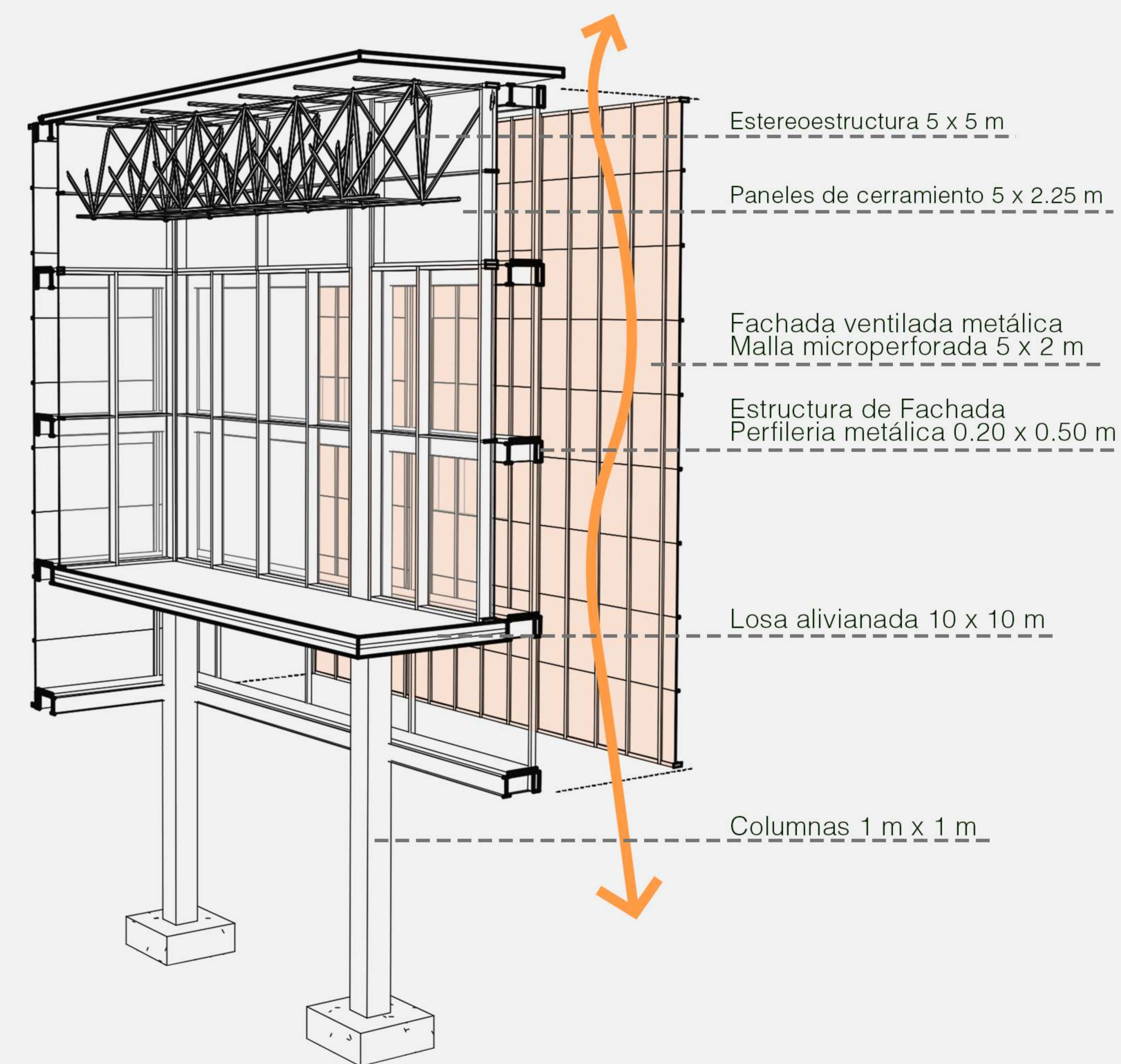
VISTA SUDOESTE
