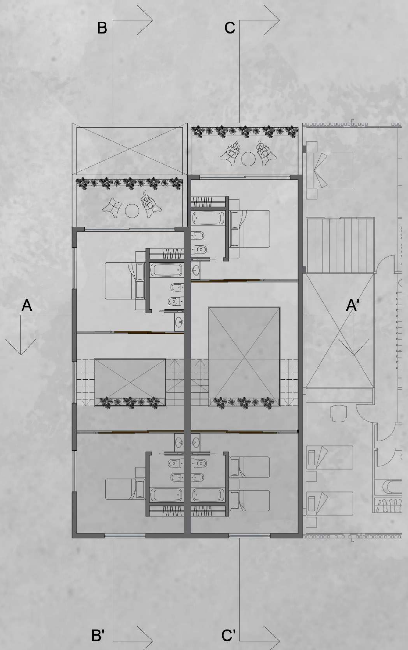
PLANTA NIVEL 2
